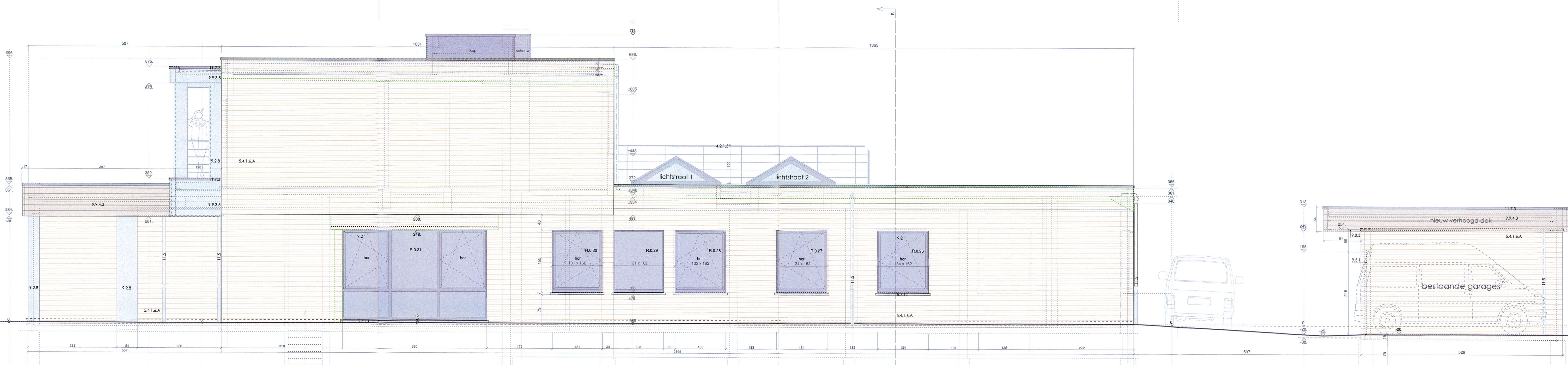
ZIJGEVEL RECHTS zuid oost schaal 1/50
