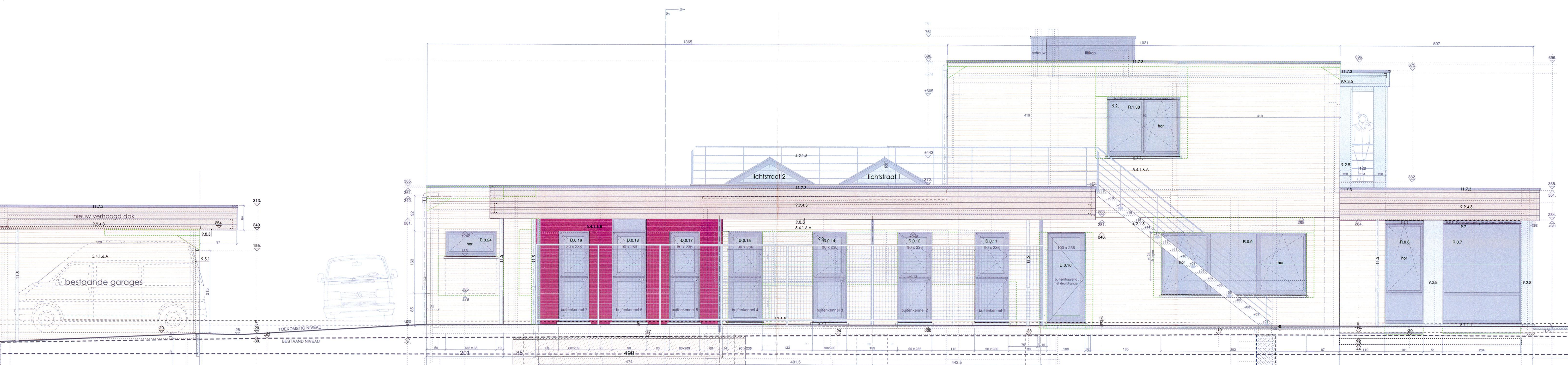
ZIJGEVEL LINKS noord west schaal 1/50
